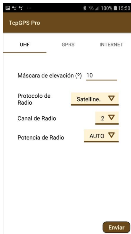
Figura 3. Modo de trabajo Rover UHF
